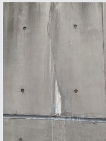
擁壁の漏水
